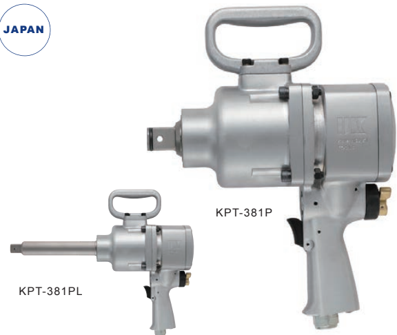
KPT-381P 1" Sq Drive KPT-381PL w/ 8" Long Anvil
